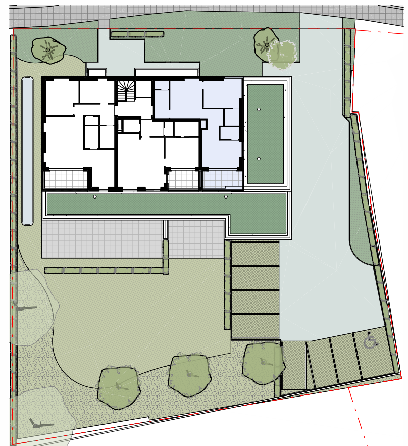
Inplantingsplan, schaal 1/400
